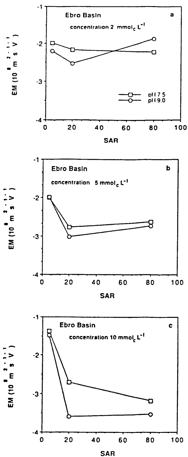
Figura 5.- Movilidad electroforética en relación con SAR, pH y concentración salina para la arcilla del suelo de la Cuenca del Ebro.
