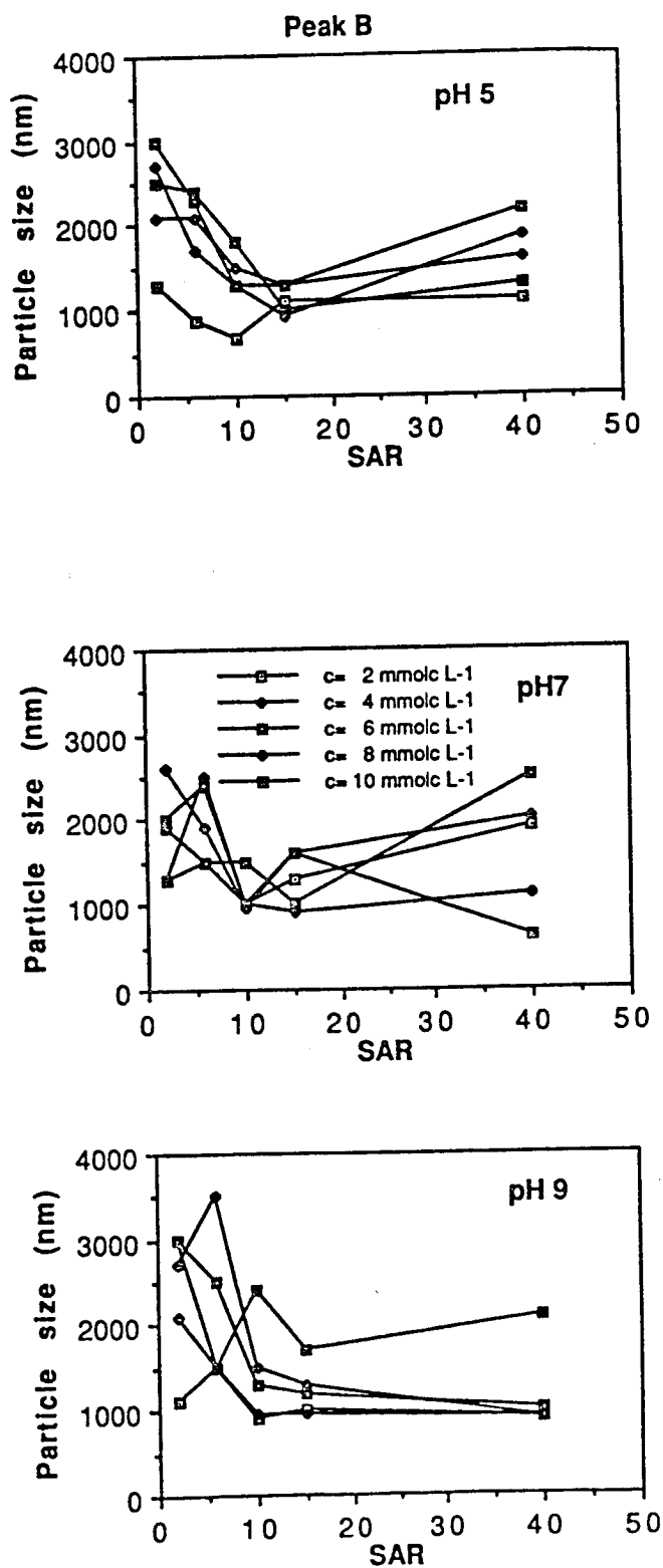
Figura 4.- Cambios en el tamaño de partícula de los dominios de Silver Hill Illita con SAR, concentración salina y pH.
