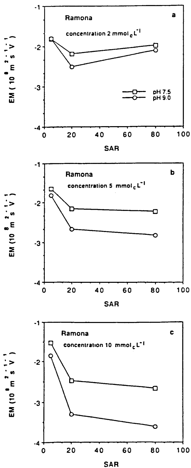
Figura 6.- Movilidad electroforética en relación con SAR, pH y concentración salina para la arcilla del suelo Ramona.
