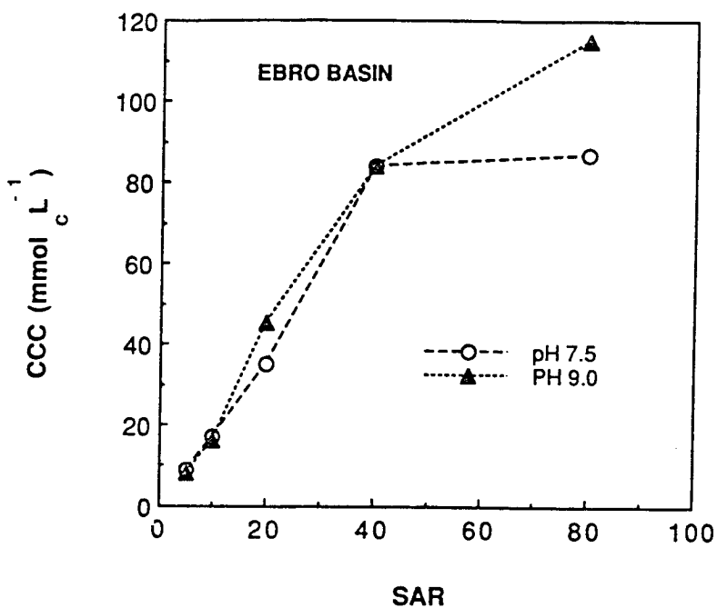
Figura 1.- Valores medios de la concentración crítica de coagulación (CCC) de las ocho muestras del suelo de la Cuenca del Ebro en función del SAR y pH. Errores standard están indicados.
