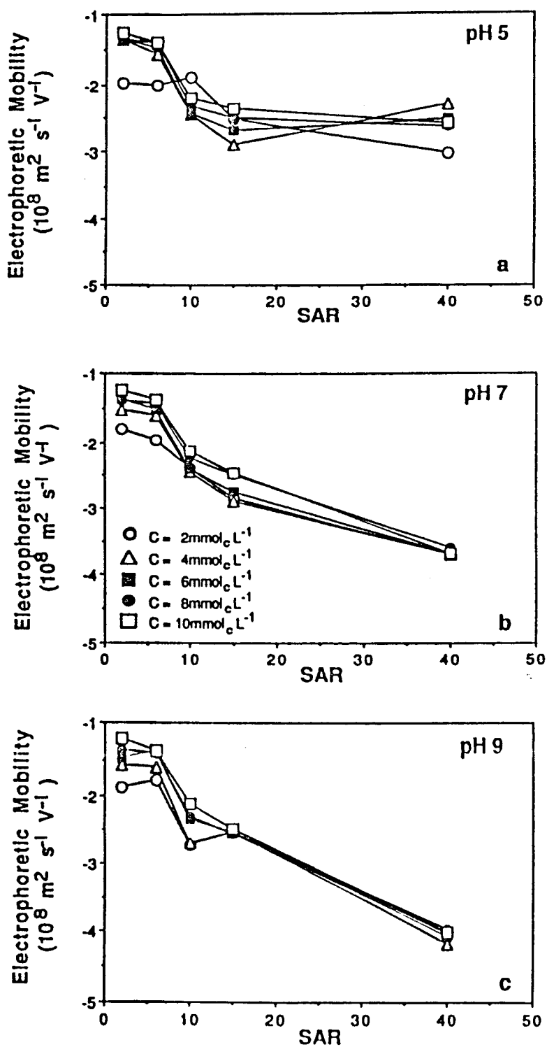
Figura 7.- Movilidad electroforética en relación con SAR, pH y concentración salina para la Silver Hill IIita.
