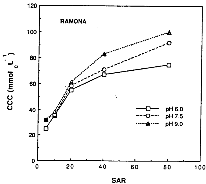
Figura 2.- Valores medios de la concentración crítica de coagulación (CCC) de las dieciseis muestras del suelo Ramona en función del SAR y pH. Errores standard están indicados.
